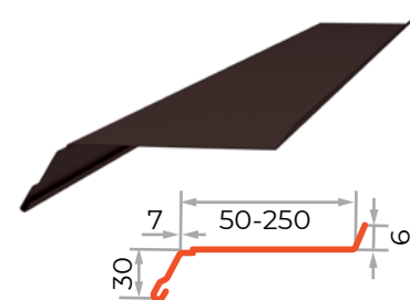
Отлив оконный
