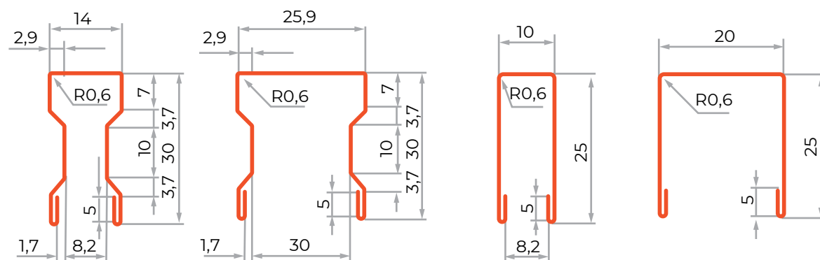
Планка фигурная для забора C8, C20, C21
